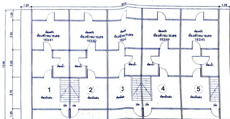
แปลนพื้นที่ล่าง อาคารชั้นนายร้อย ขนาด 5 ครอบครั้ว อาคารหมายเลข 179
