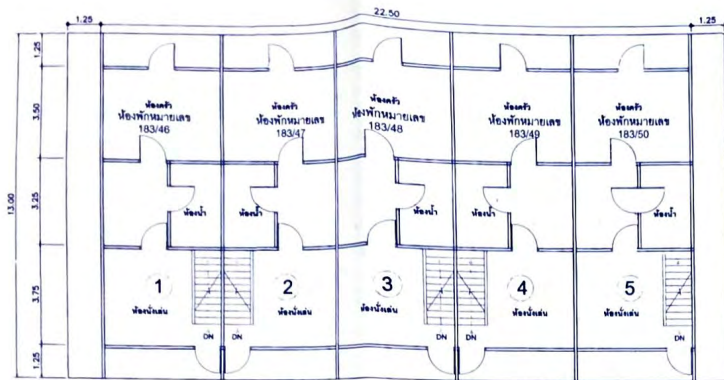
แปลนพื้นที่ล่าง อาคารชั้นนายร้อย ขนาด 5 คกรบควัว อาคารหมายเลข 180
