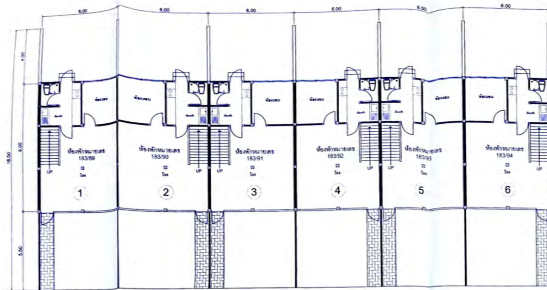
แปลนพื้นที่ชั้นล่าง อาคารชั้นนายพัน ขนาด 6 ครอบครั้ว อาคารหมายเลข 176
