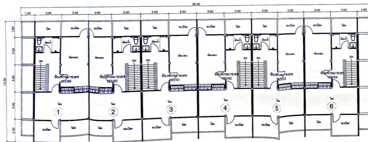
แปลนพื้นที่ชั้นล่าง อาคารชั้นนายพัน ขนาด 6 ครอบครั้ว อาคารหมายเลข 176
