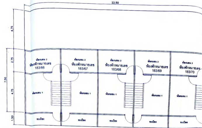
แปลนพื้นชั้นบน อาคารชั้นนายร้อย ขนาด 5 คอปรควิว อาคารหมายเลข 184
