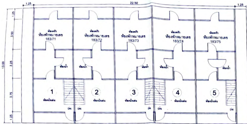
แปลนพื้นที่ล่าง อาคารชั้นนายร้อย ขนาด 5 ครอบครั้ว อาคารหมายเลข 185
