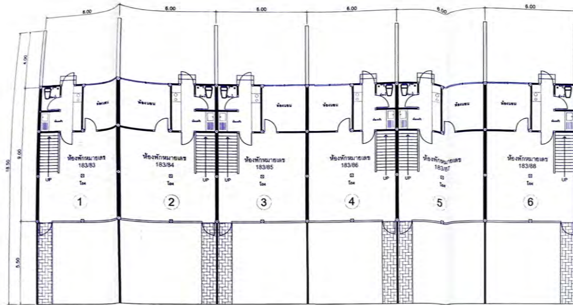
แปลนพื้นชั้นล่าง อาคารชั้นนายพัน ขนาด 6 ครอบครั้ว อาคารหมายเลข 175 SCALE 1:100
