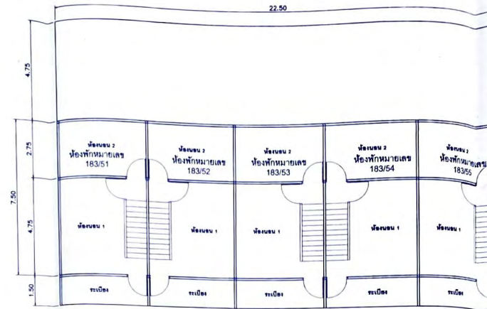
แปลนพื้นที่บน อาคารชั้นนายร้อย ขนาด 5 ครอบครัว อาคารหมายเลข 181
