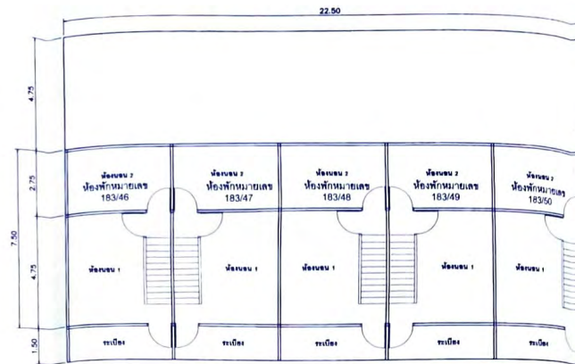
แปลนพื้นที่บน อาคารชั้นนายร้อย ขนาด 5 คกรบควัว อาคารหมายเลข 180
