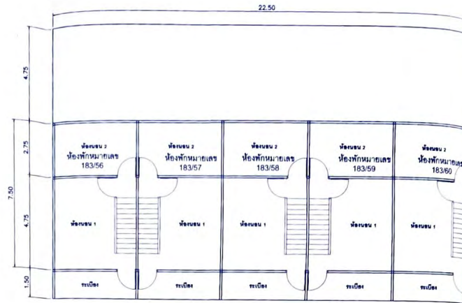
แปลนพื้นชั้นบน อาคารชั้นนายร้อย ขนาด 5 คออบคิ้ว อาคารหมายเลข 182 SCALE 1:100
