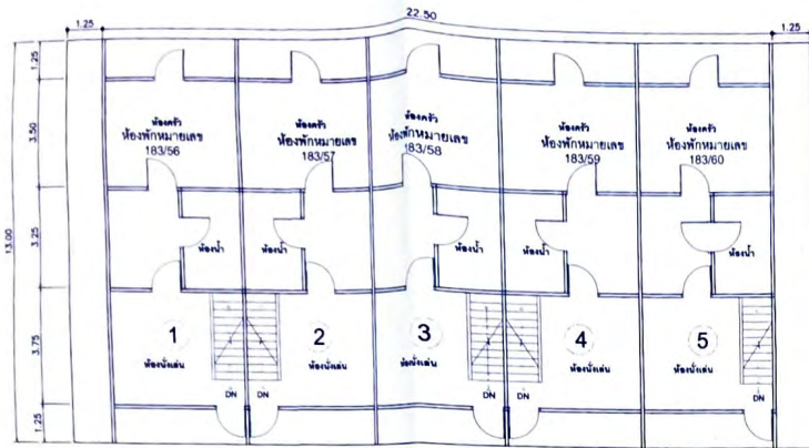
แปลนพื้นชั้นล่าง อาคารชั้นนายร้อย ขนาด 5 คออบคิ้ว อาคารหมายเลข 182 SCALE 1:100
