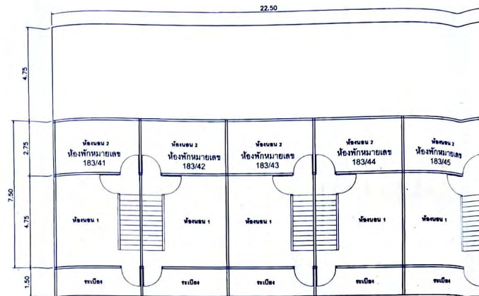
แปลนพื้นที่บน อาคารชั้นนายร้อย ขนาด 5 ครอบครั้ว อาคารหมายเลข 179
