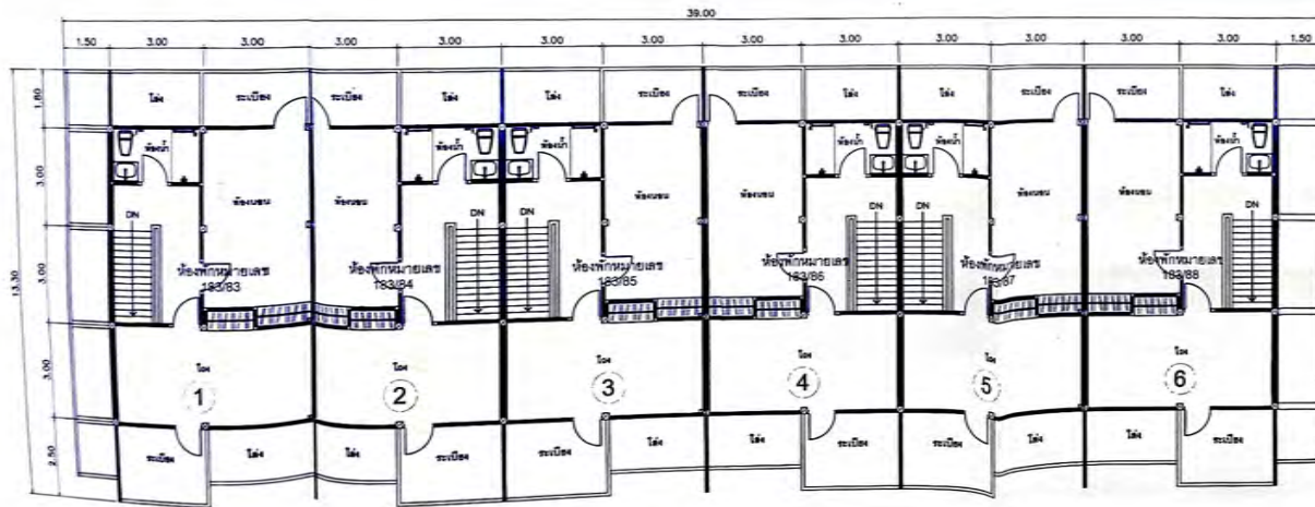
แปลนพื้นชั้นล่าง อาคารชั้นนายพัน ขนาด 6 ครอบครั้ว อาคารหมายเลข 175 SCALE 1:100
