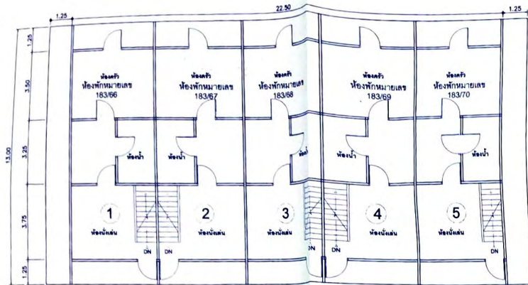
แปลนพื้นชั้นล่าง อาคารชั้นนายร้อย ขนาด 5 คอปรควิว อาคารหมายเลข 184
